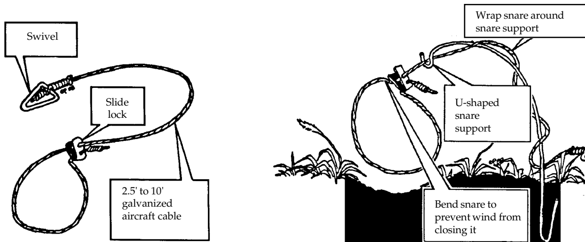
Fig. 31. Coyote snare
